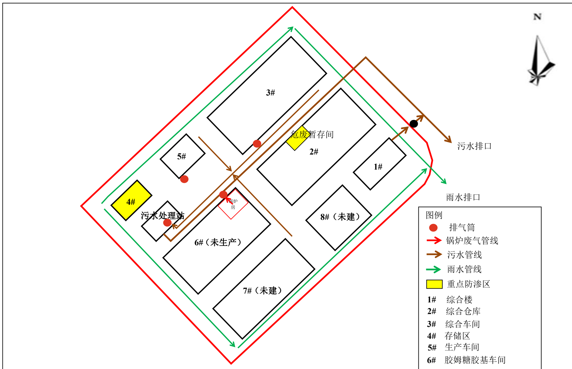
附图3 项目厂区平面布置图、雨污管网图和分区防渗图
